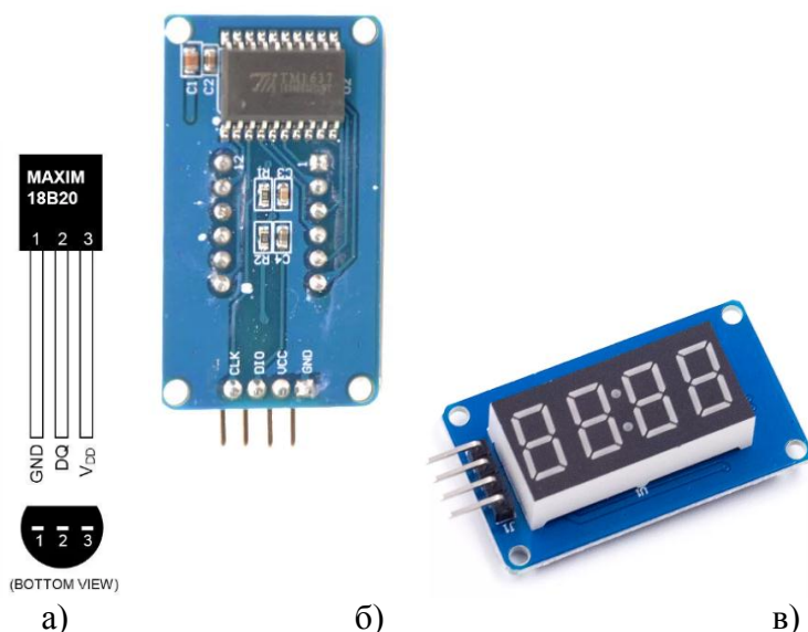
Рисунок 2 – Используемые микросхемы
